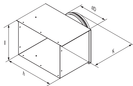
Вертикальний адаптер
