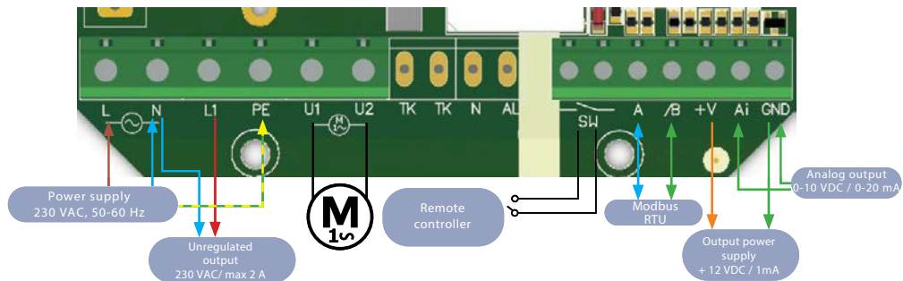
Рис. 3. Електрична схема
