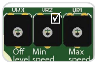
Рис. 7. Тример мін. швидкості
