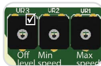
Рис. 8. Тример налаштування рівня вимкнення
