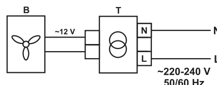
ТРФ-220/12-25 КТР
