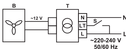
ТРФ-220/12-25 КТ/КТН
