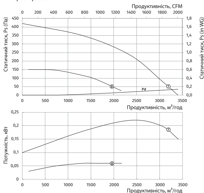
Типорозмір: 355
