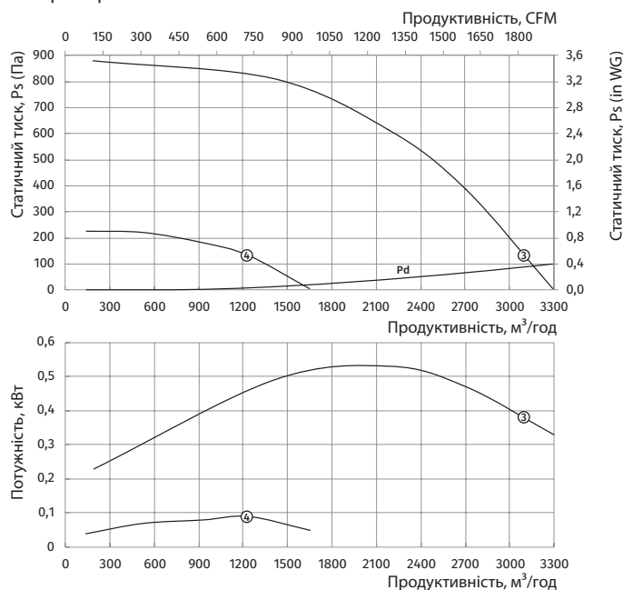
Типорозмір: 280
